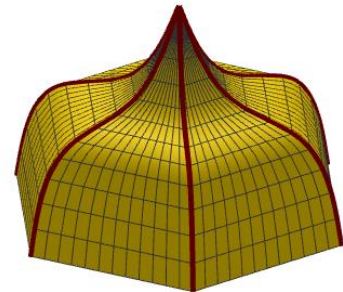
Imagen 22. Cúpula construida mediante curvas Spline y superficies regladas.
