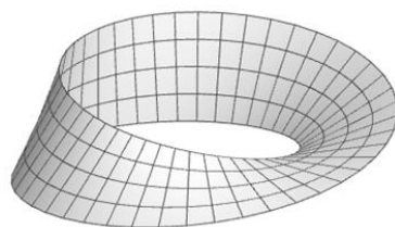
Imagen 13. Banda de Moebius.
