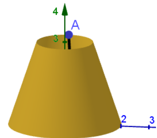
Imagen 3. Tronco de cono como superficie de revolución de un segmento.
