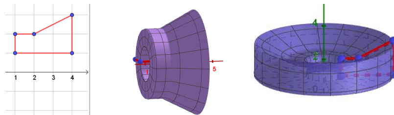
Imagen 5. Superficies de revolución de un polígono.
