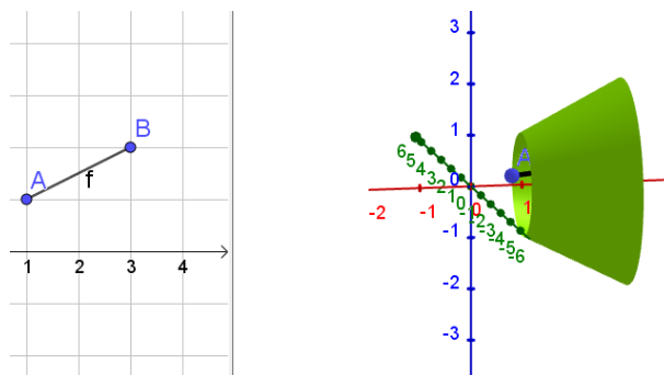
Imagen 2. Superficie de revolución de un segmento alrededor del eje x
