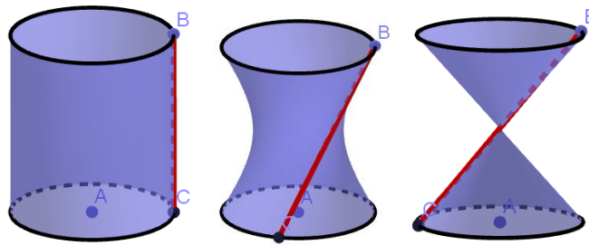
Imagen 4. Cilindro, hiperboloide de una hoja y cono como superficies de revolución de un segmento.
