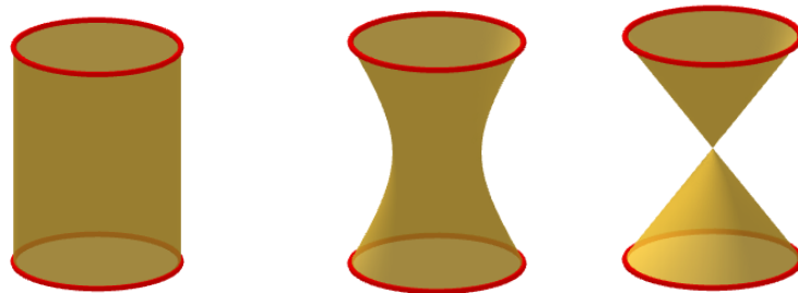
Imagen 19. Cilindro, hiperboloide y cono contruidos como superficies regladas entre dos circunferencias.
