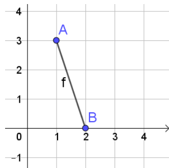
Imagen 3. Tronco de cono como superficie de revolución de un segmento.
