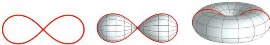
Imagen 14. Lemniscata de Bernoulli y superficies al girar sobre eje x e y respectivamente.
